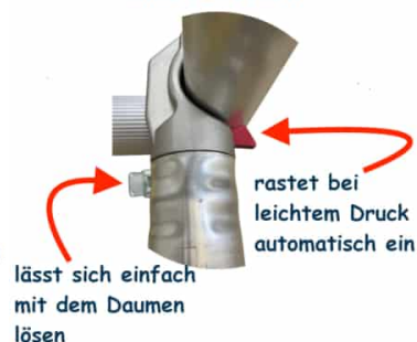
Streben-Rahmenverbindung ohne Schrauben
