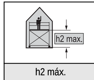
Altura máxima admissível do andaime, quando utilizado dentro de edifícios:
