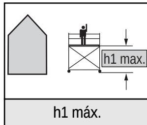
Altura máxima admissível do andaime, quando utilizado fora de edifícios:
