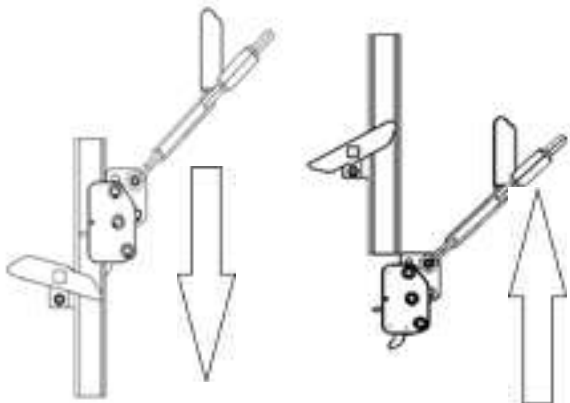
Abb. 17 Einstieg in die Steigschutzeinrichtung
